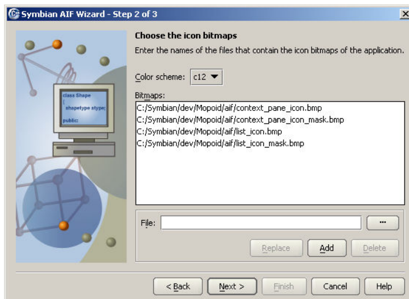
تصویر ۳: اضافه کردن آیکن‌ها به برنامه
